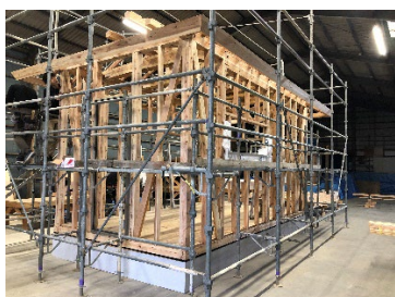
現地施工試験体
