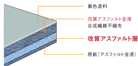
改質アスファルトフェルトイメージ図
